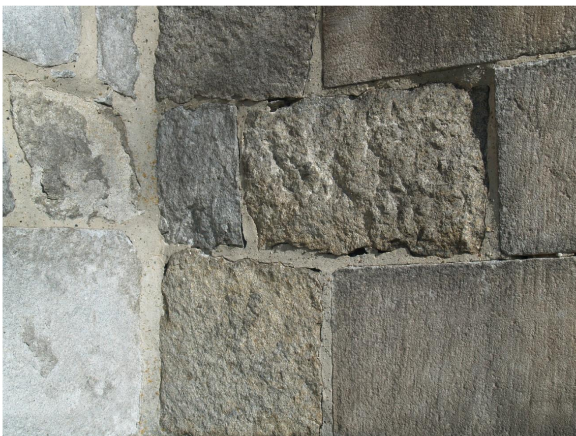
Rysunek 8. Ściana Mauzoleum wykonana z kamienia łupanego i ciosanego. Po lewej stronie granit, po prawej piaskowiec.
